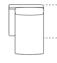
penisola da 114 dx/sx L. 114 P. 160 H. 88
